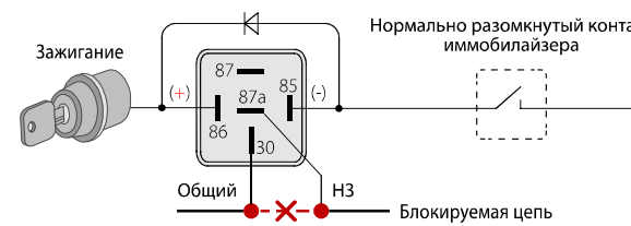
Подключение внешнего реле блокировки
